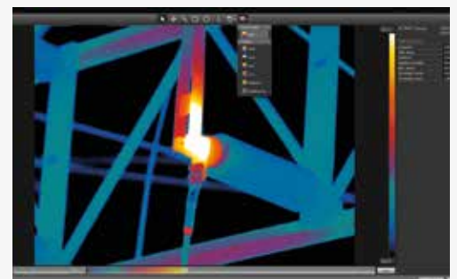
FLIR Tools+ permet d'ajuster les images en changeant de palette et en modifiant des paramètres comme l'émissivité, la température réfléchie, etc.
