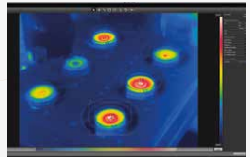
FLIR Tools+ vous permet d'éditer les images radiométriques. Vous pouvez aussi ajouter des outils de mesure perfectionnés tels que des points, des zones rectangulaires, des zones circulaires, des lignes et Delta T.
